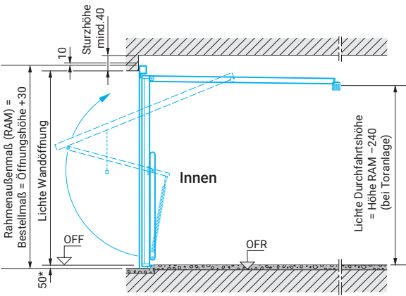
Vertikalschnitt
