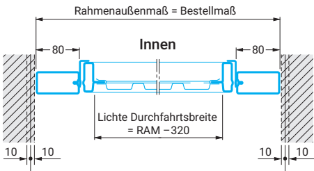
Einbau in der Öffnung
