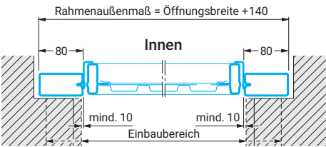
Einbau hinter der Öffnung
