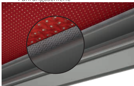
4 tracfix Tuchführung – ohne Spalt zur Führungsschiene 1)
