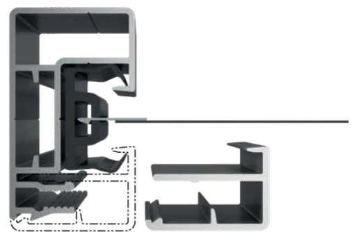
Befestigung an markilux construct
